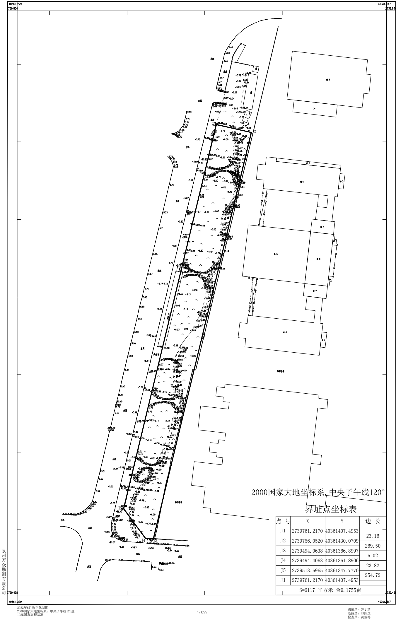
石狮市华侨中学扩建用地勘测定界图
