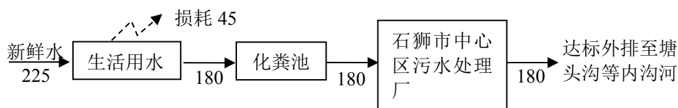
图2.8-1 项目水平衡图(单位: t/a)
