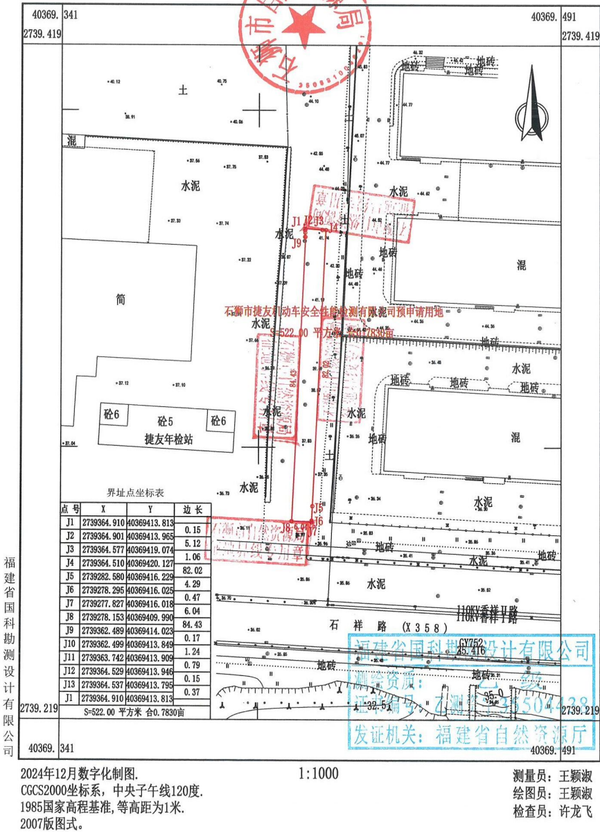
石狮市捷友机动车安全性能检测有限公司预申请用地勘测界定图 2739.22-40369.34
