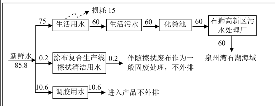
图2.8-1 项目水平衡图（单位：t/a）
