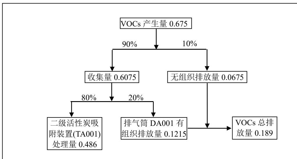
图 2.8-2 项目 VOCs 物料平衡图 (t/a)
