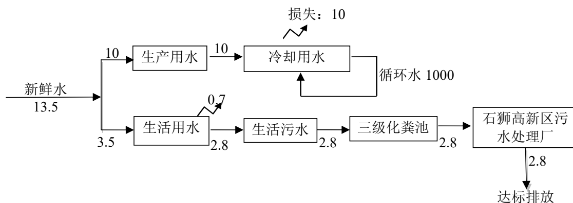
图 2.7-1 项目水平衡图 (单位: t/d)
